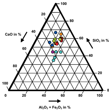
Dreistoffdiagramm für die Hauptbestandteile untersuchter MV-Aschen
