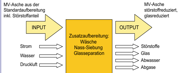
Skizze zur Input-Output-Analyse für eine mögliche zusätzliche Aufbereitung der MV-Asche zur Störstoffreduzierung
